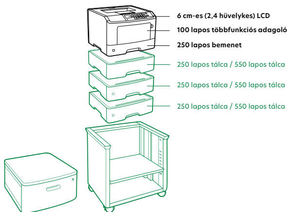
Állítható nyomtatóállvány
